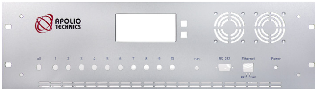
Frontplatte aus eloxiertem Aluminium, Größe: 483,00 x 132,50 mm Diese Frontplatte können Sie herunterladen
